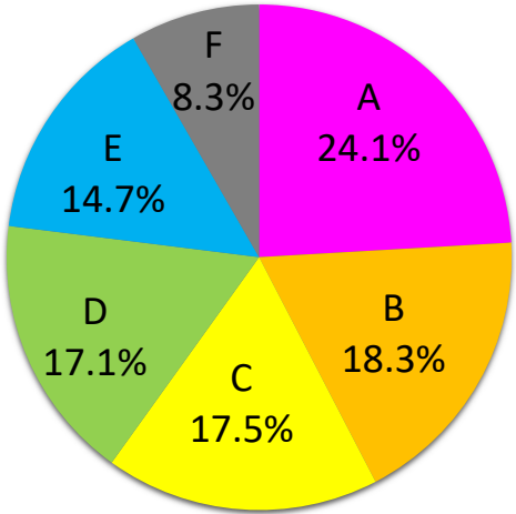
格付分布
