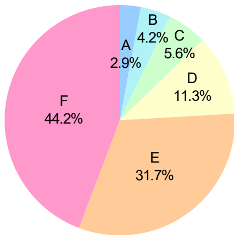
図表A 第 22 回「格付ロジック改定によるRM格付変動の影響」／生存企業の格付分布
