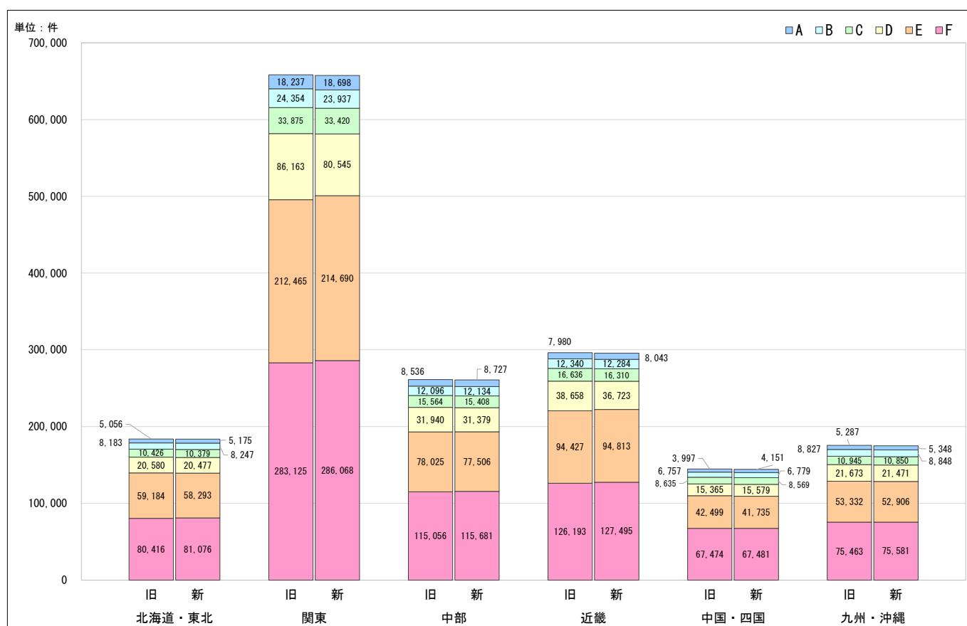
図表D 第22回「格付ロジック改定によるRM格付変動の影響」／
