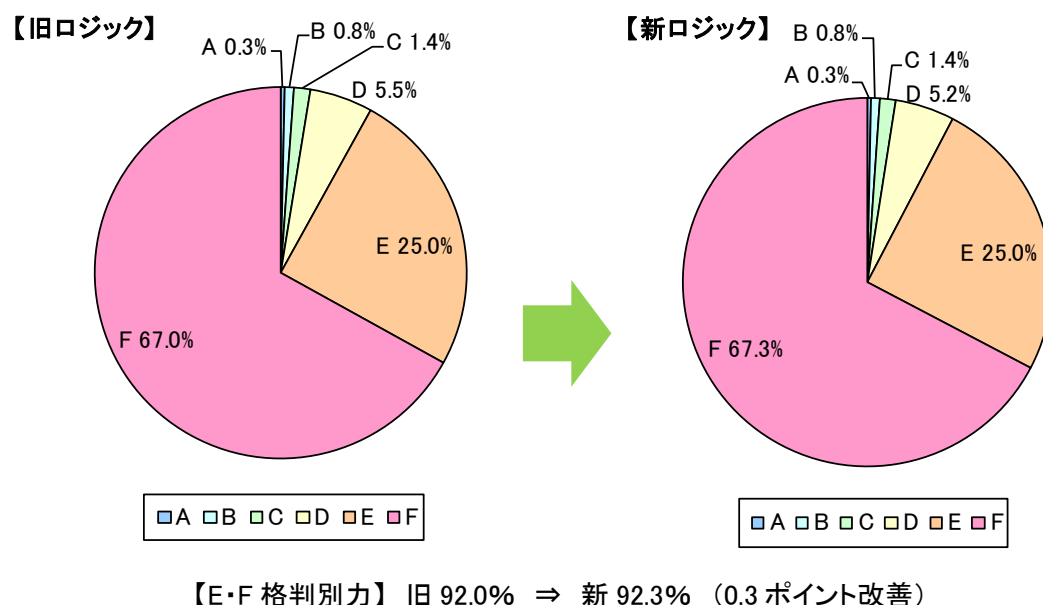
図表D 第22回「格付ロジック改定によるRM格付変動の影響」／
